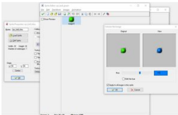
Sprites färben.
